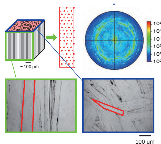
■多結晶中の単結晶の弾性特性を解析するための新手法
