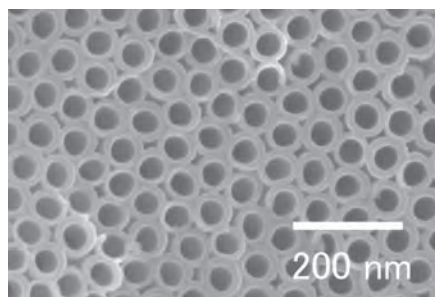
■電気化学的手法により生成する酸化チタン・ナノホール・アレイ
