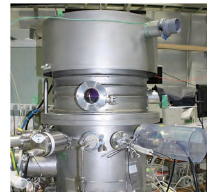
■sugimoto1-IMG_9034ts: プラズマプロセス装置
