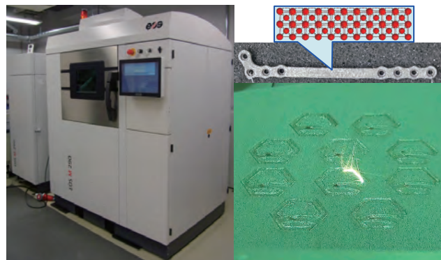
■3Dプリンタによる新たな生体材料の創製。形状だけでなく、材質（原子配列など）・機能の制御が可能になります。
