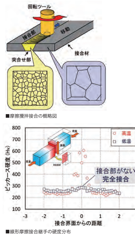
■線形摩擦接合継手の硬度分布
