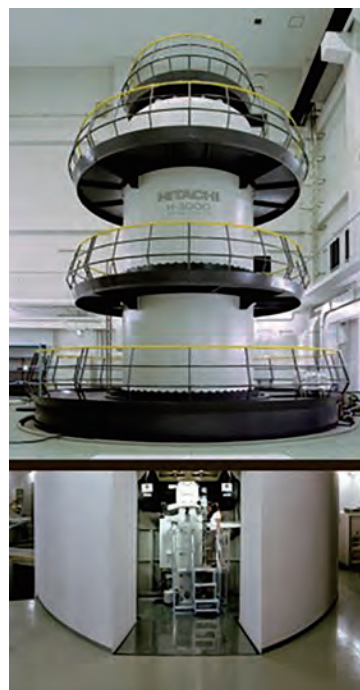
■300万ボルト超高圧電子顕微鏡
