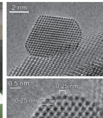
■触媒として気体分子と相互作用している金属ナノ粒子
