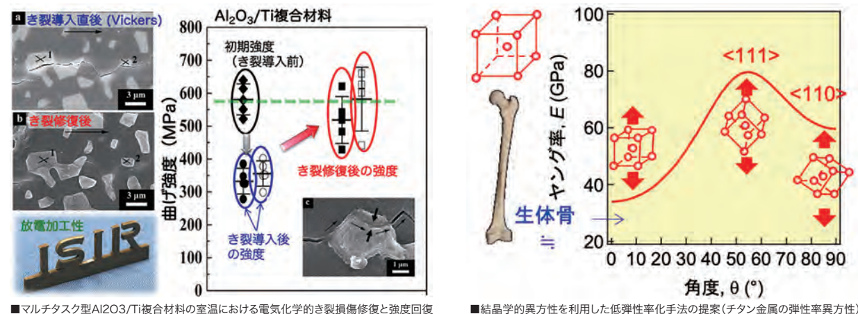
■マルチタスク型 \text{Al}_2\text{O}_3/\text{Ti} 複合材料の室温における電気化学的き裂損傷修復と強度回復
