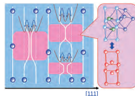
■チタン合金において発見した新たな相転移
