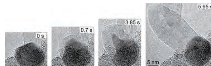
■カーボンナノチューブの核形成と成長のその場観察
