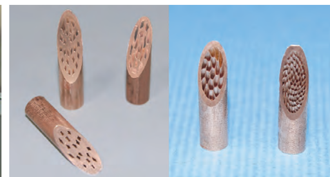
■固相接合を用いた新加工プロセスによる高強度ポラス鋼
